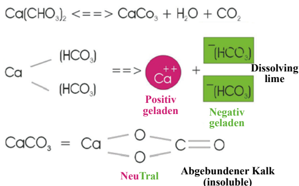
Bild 7: Schematische Darstellung von gelöstem und abgebundenem Kalk
