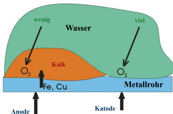
Bild 12a: Korrosion durch unterschiedlich dicke Kalkablagerungen
