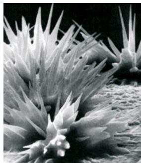
Bild 10: Kristallbildung in einer Phosphatschutzschicht
