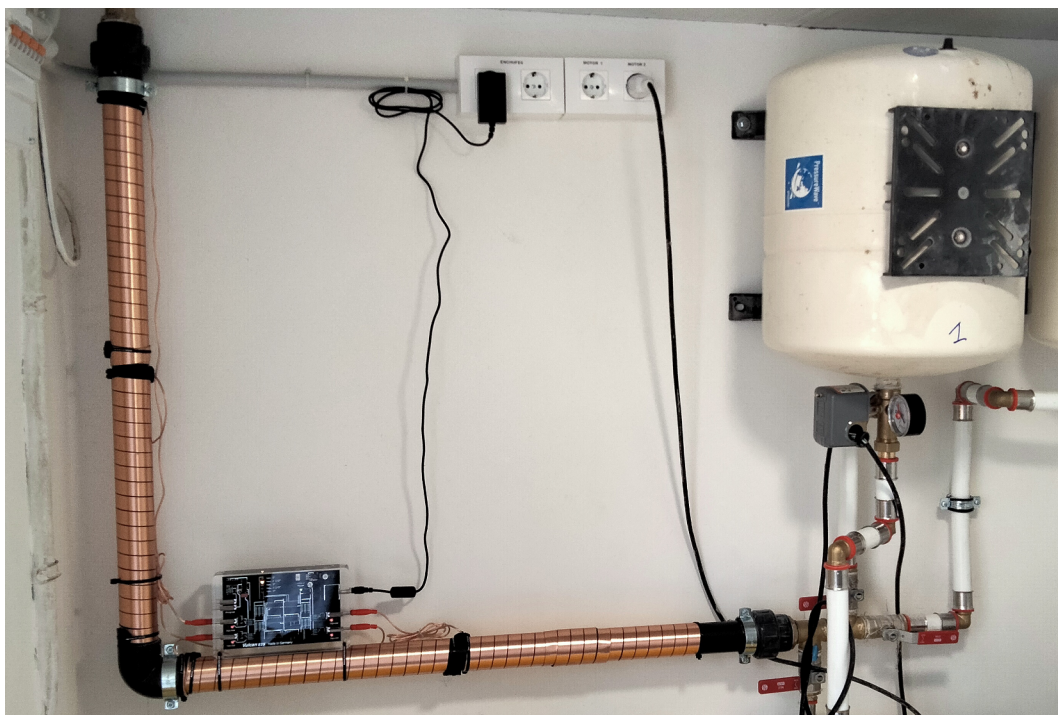
Vulcan S25 Kaltwasser Hauptleitung mit Ø 50 mm
