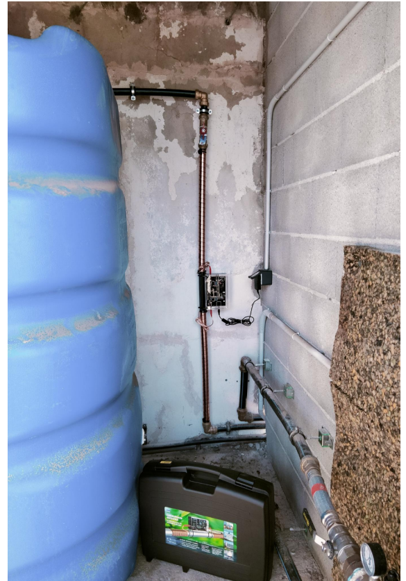
Vulcan S10 Kaltwasser Hauptleitung mit Ø 19 mm
