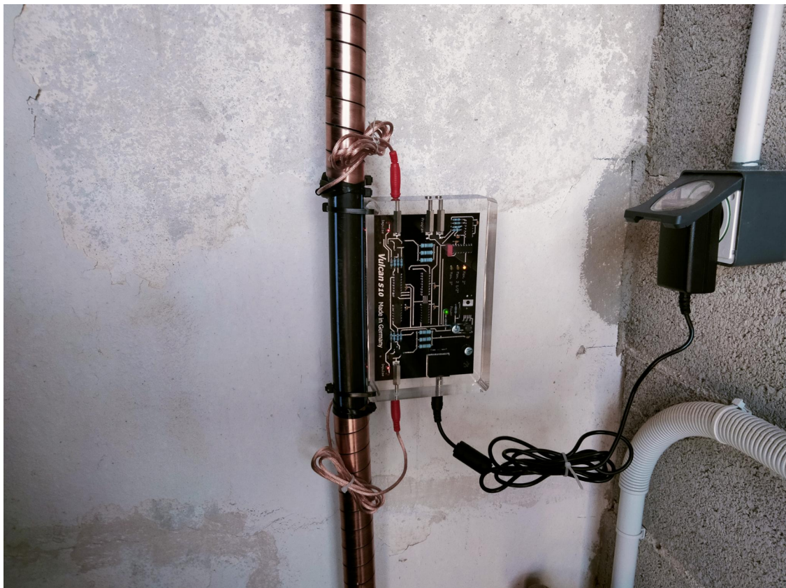
Vulcan S10 Kaltwasser Hauptleitung mit Ø 19 mm
