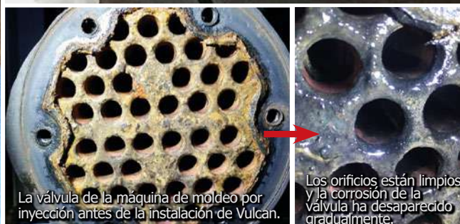
Vulcan S150 se instaló en la tubería del taller libre de polvo para tratar el agua de la máquina de moldeo por inyección.
