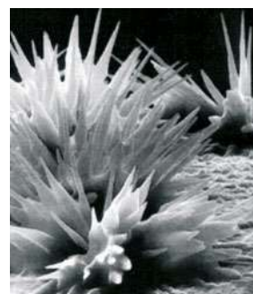
Fig. 10: Capa protectora de fosfato
