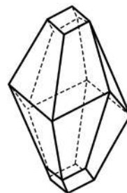
Fig. 2: Célula elemental de una calcita (sistema trigonal)
