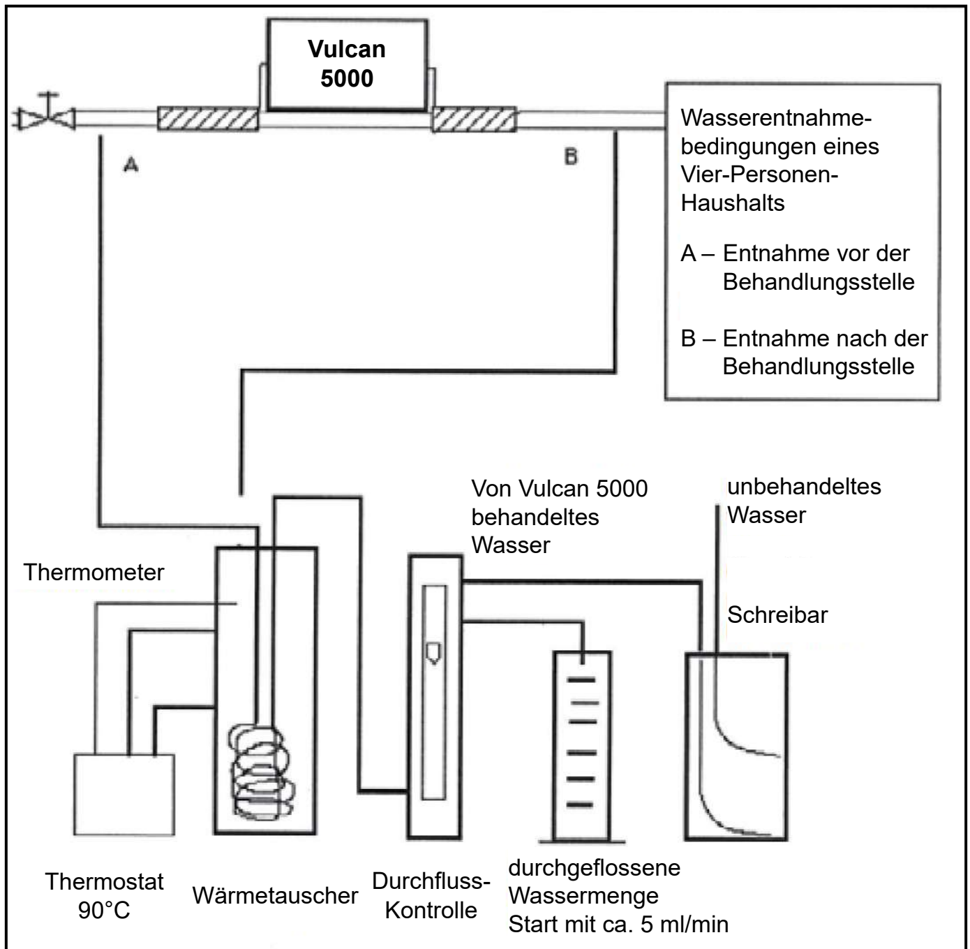
Schema für den Funktionsnachweis des Wasseraufbereitungsgerätes Vulcan 5000 (In der Schemazeichnung ist nur einer der beiden Prüfungen aufgeführt)
