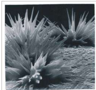
Bild 10: Kristallbildung in einer Phosphatschutzschicht
