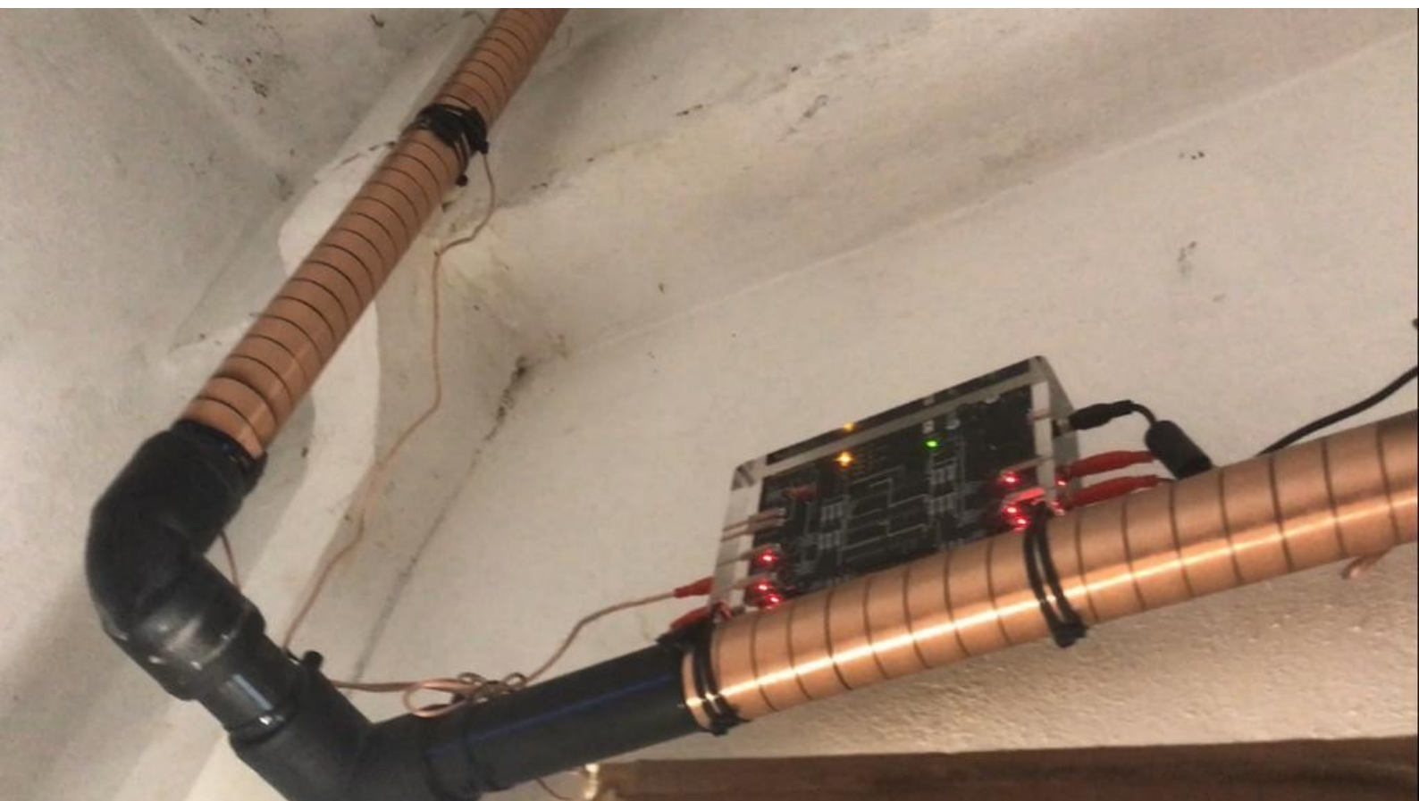
Vulcan S25 en el tubo general de agua fría
