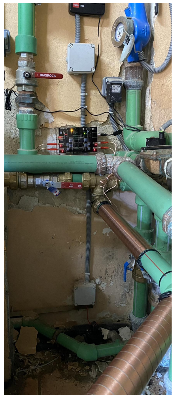
Vulcan S50 an der Kaltwasserleitung mit Ø 63 mm
