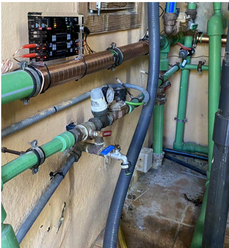
Vulcan S50 en el tubo de agua fría con Ø 63 mm
